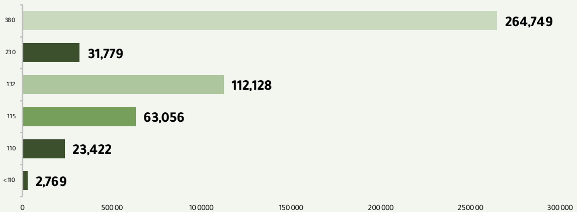
سعة محوّلات النقل حسب الجهد
