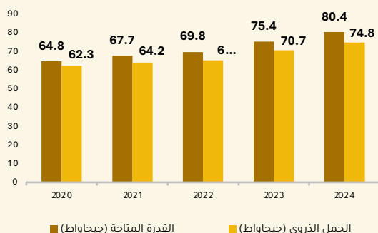
الحمل الذروي والقدرة المتاحة 2020-2024
