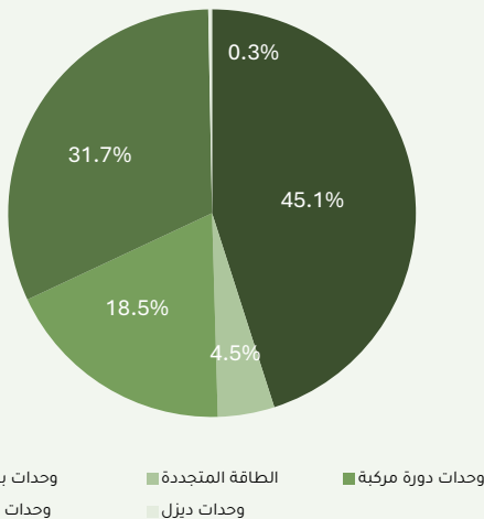
توزيع السعة حسب نوع الوحدة 2024
